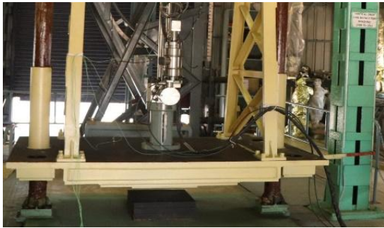
Vibration Stand
